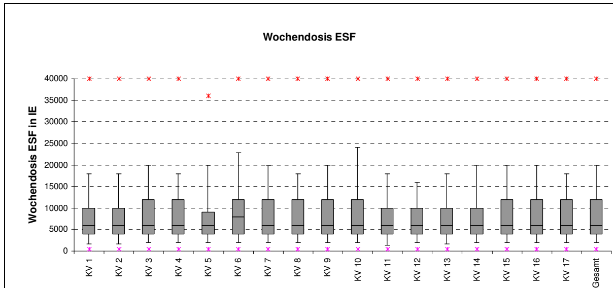
Abbildung 15: Wochendosis ESF
