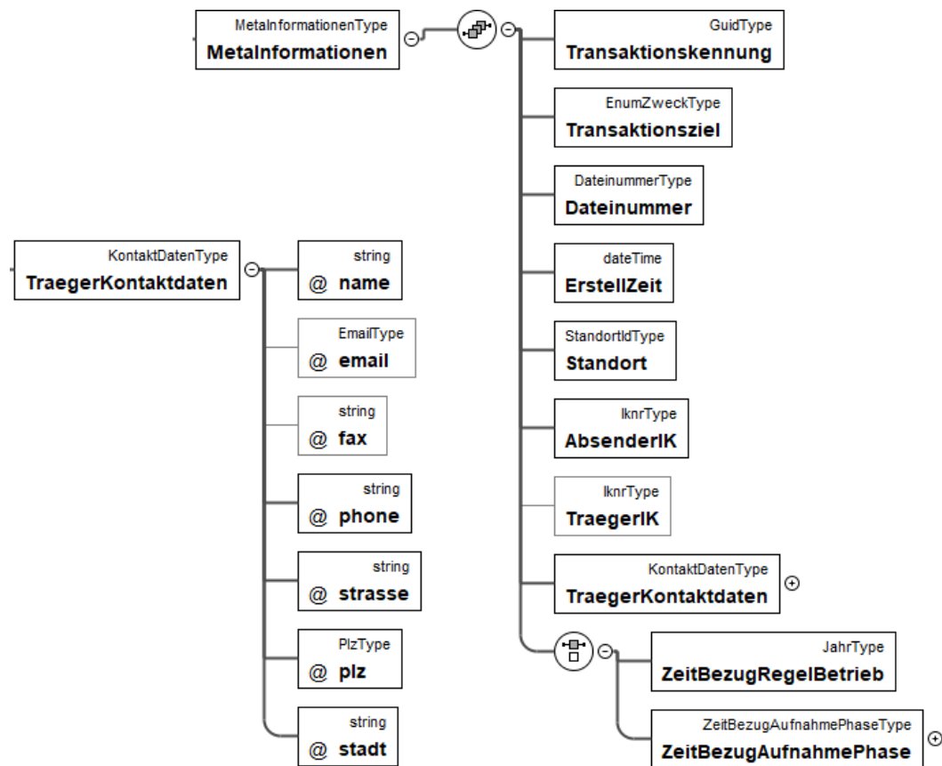
Abbildung 6: XML-Schema zur Übermittlung der Leistungsmengen – Metainformationen Details
