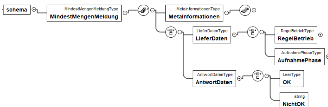
Abbildung 5: XML-Schema zur Übermittlung der Leistungsmengen – Metainformationen und Lieferdaten
