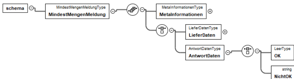
Abbildung 9: XML-Schema zur Übermittlung der Antwort von den Landesverbänden der Krankenkassen an den Leistungserbringer
