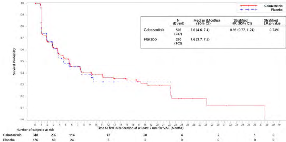
Abbildung 1: Kaplan-Meier-Kurven zum Gesundheitszustand (EQ-5D VAS), Zeit bis zur Verschlechterung um \geq 7 Punkte
