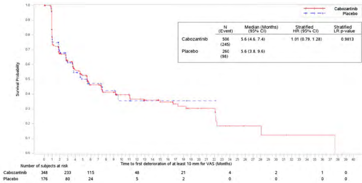
Abbildung 2: Kaplan-Meier-Kurven zum Gesundheitszustand (EQ-5D VAS), Zeit bis zur Verschlechterung um \geq 10 Punkte
