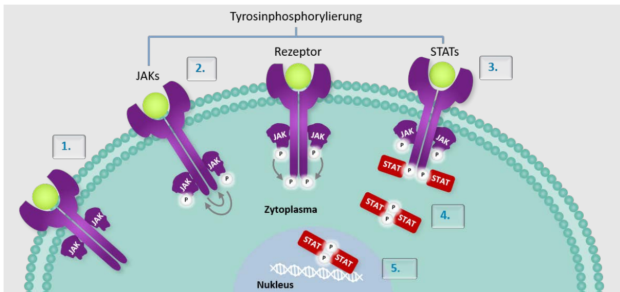
Abbildung 1: JAK-STAT-Signalweg
