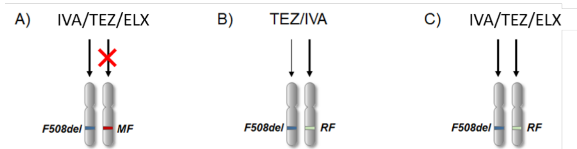
Abbildung 3-4: Wirkprinzipien der Tripel-Kombination Ivacaftor/Tezacaftor/Elxacaftor und Tezacaftor/Ivacaftor bei verschiedenen Mutationskombinationen:
