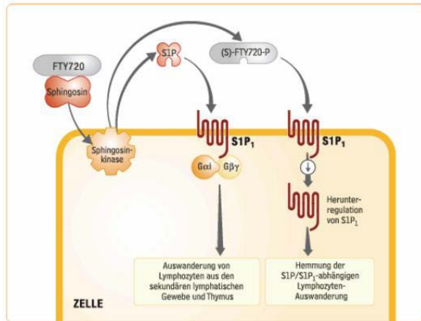
Abbildung 2-1: Zelluläre Effekte von Fingolimod und S1P; aus Chiba et al., 2005 (21)
